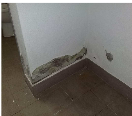
Umidità ascendente lungo il perimetro dei muri
