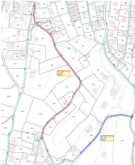
(Progetto Rosso in fase di realizzazione Via Prelongo) Progetto Blu Via Selvaccia oggetto RT
